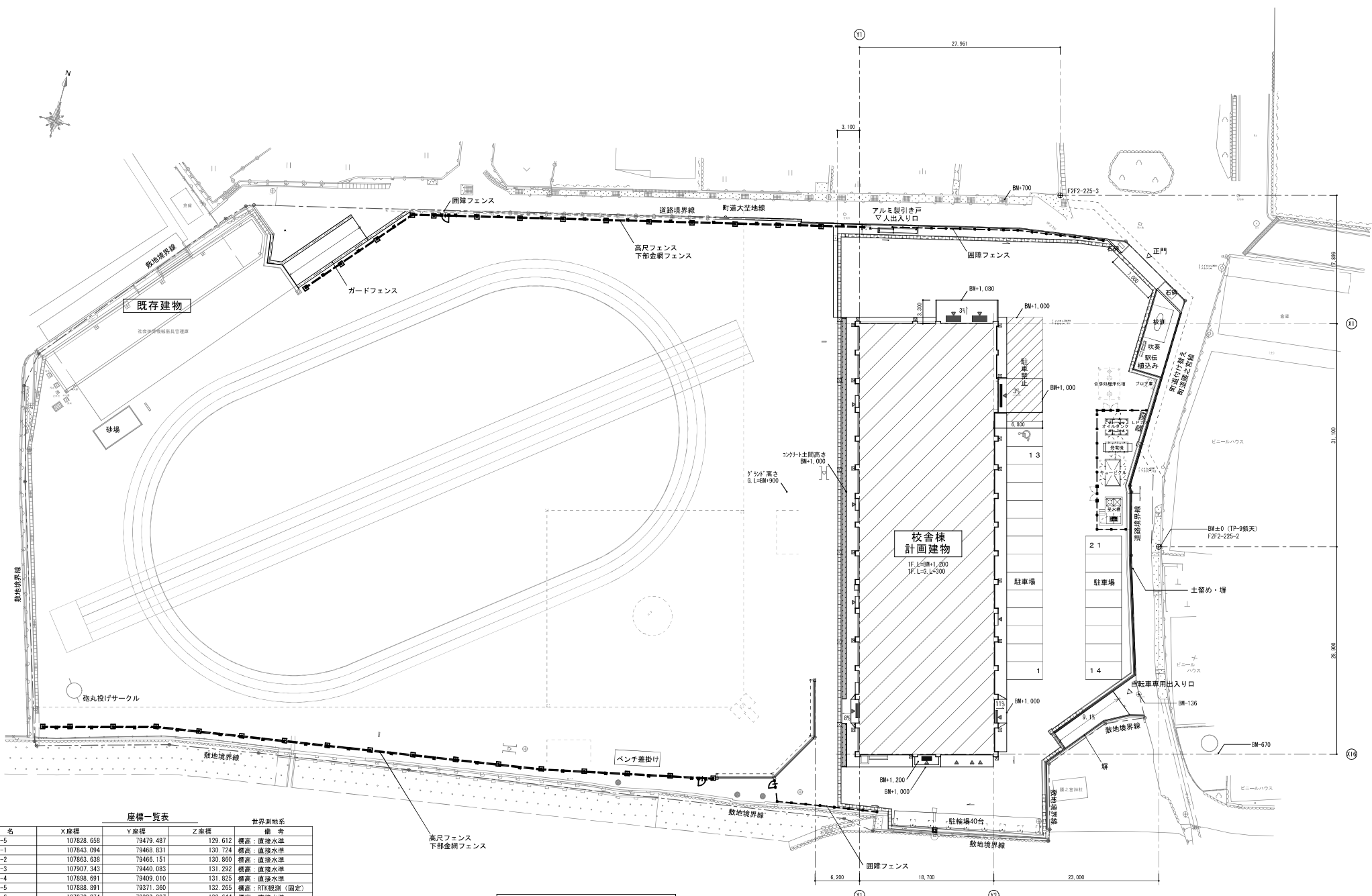
配置図（整備後） A1 : 1/250
